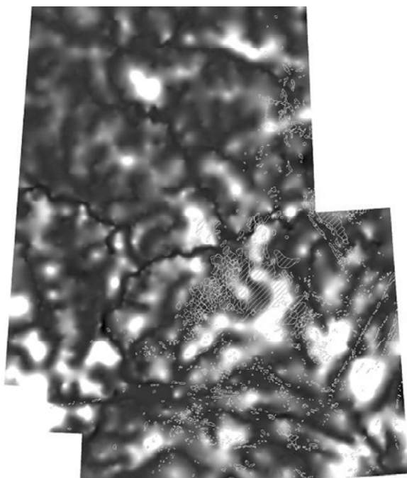
Рис. 7. Наложение карты разности базисных поверхностей 5-го и 6-го порядков и карты месторождений нефти
