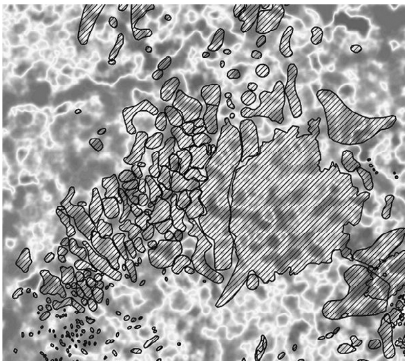
Рис. 9. Осредненный показатель макротрещиноватости осадочного чехла и расположение месторождений нефти (юго-восток Республики Татарстан)
