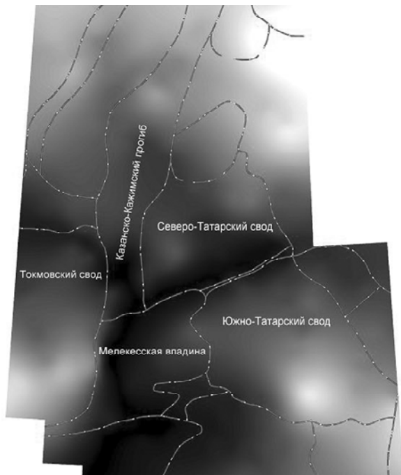
Рис. 2. Сопоставление базисной поверхности 7-го порядка с известными тектоническими элементами
