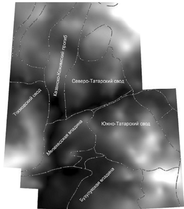
Рис. 3. Сопоставление базисной поверхности 6-го порядка с известными тектоническими элементами
