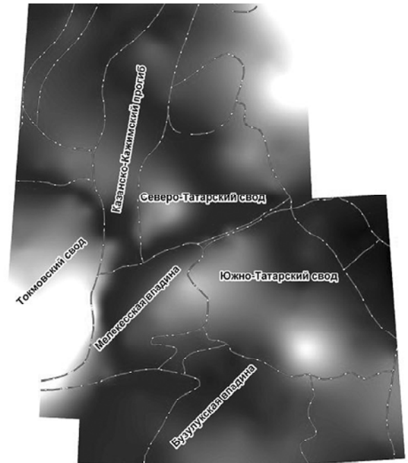
Рис. 5. Наложение тектонических элементов I порядка на разность базисных поверхностей 7-го и 8-го порядков
