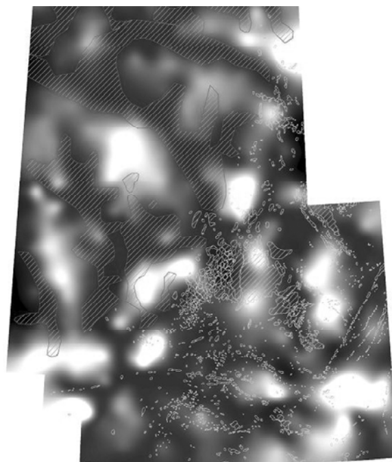
Рис. 8. Наложение карты разности базисных поверхностей 6-го и 7-го порядков и карты месторождений нефти
