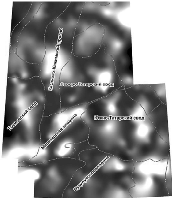
Рис. 4. Наложение тектонических элементов I порядка на разность базисных поверхностей 6-го и 7-го порядков
