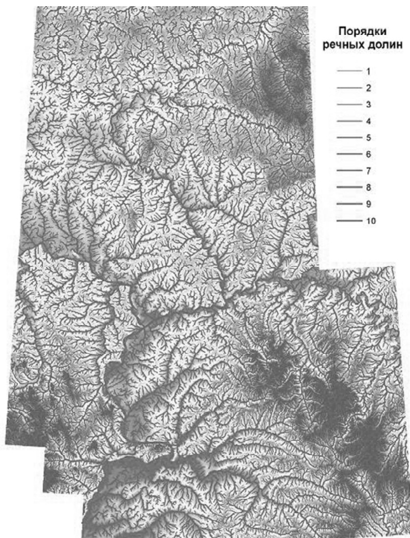
Рис. 1. Цифровая модель рельефа и геометрическая сеть речных долин
