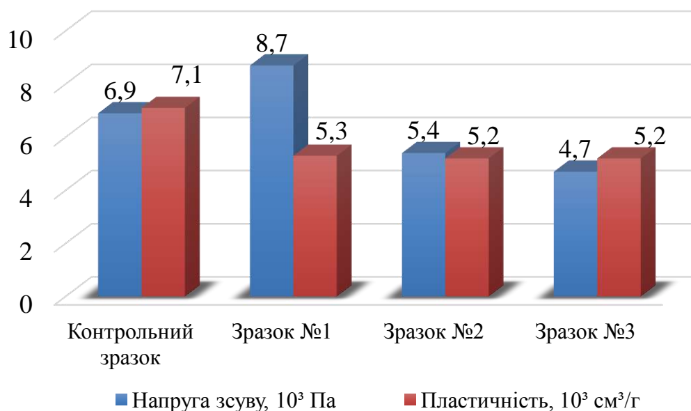
Рис. 2. Зміна граничної напруження зсуву та пластичності у дослідних зразках
