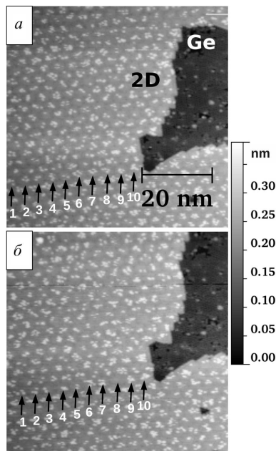
Рис. 4. Два послідовних СТМ-зображення, одержаних на одній ділянці поверхні Ge(111) площею 62 \times 62 нм, що включає значну ділянку, вкриту 2D поверхневим шаром. Помітно невеликий зсув між зображеннями (а) та (б), внаслідок термодрейфу та артефактів п'езосканера СТМу. Тунельна напруга на зразку – 2,5 В, тунельний струм 0,3 нА. 10 одних і тих самих вузлів суперґратки промарковано нумерованими стрілками
