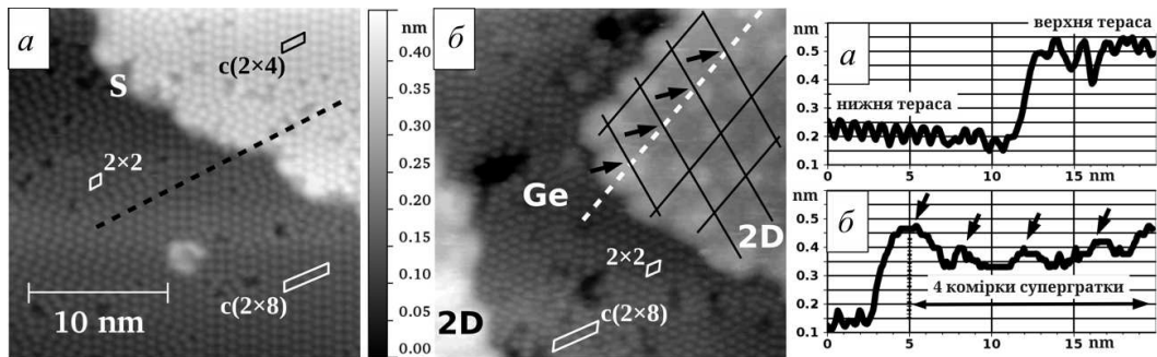
Рис. 2. СТМ-зображення із атомною роздільною здатністю (поле зору 25 \times 25 нм): a – чиста реконструйована поверхня Ge(111), тунельна напруга на зразку +2,5 В; тунельний струм 0,3 нА. Присутні структури c(2 \times 8) , c(2 \times 4) та 2 \times 2 , елементарні комірки яких промарковано відповідним чином. Одноатомну сходинку між верхньою та нижньою сусідніми терасами позначено як “S”, б – суміш чистого Ge та 2D гексагонального поверхневого шару, тунельна напруга на зразку +2 В; тунельний струм 0,3 нА, окреслено елементарні комірки 2 \times 2 та c(2 \times 8) на чистому Ge та 2D суперґратка максимумів висоти (сітка чорного кольору). Праворуч від СТМ-зображень подано поперечні перерізи висота–відстань, виміряні уздовж штрихових ліній на відповідних ділянках поверхні. Максимуми висоти на поперечному перерізі ( б ) відзначені чорними стрілками. Шкала висота–колір є спільною для обох зображень
