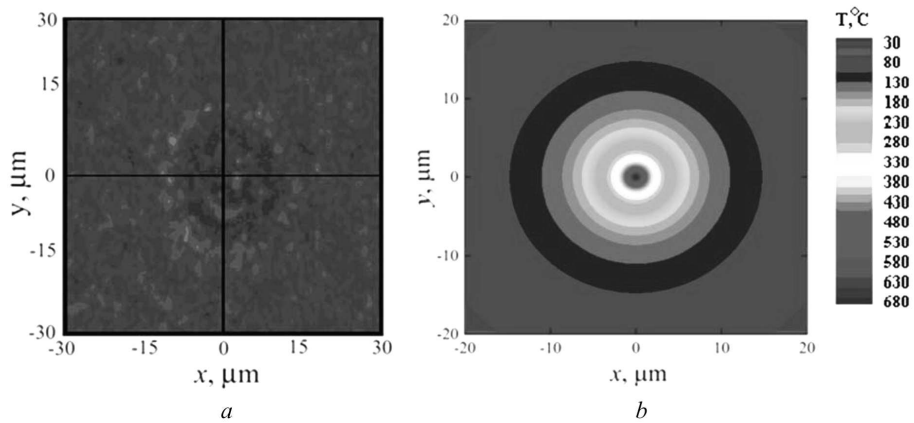
Рис. 3. Вигляд у оптичний мікроскоп сліду дії лазера збудження КРС (а); розрахунковий розподіл рівноважної температури поверхні зразка X:Y:Z = 100:100:100 нм при I = I_0 (б)
