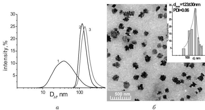
Рис. 5. ДСР визначені розміри міцел з комплексами полі(БЕП-ко-ГМА)-графт-ПЕГ та Докс (1), Les 3883 (2, 3) (полімер – 10 мг/мл, (1); [Les 3883] = 0,4 мг/мл (2); 0,8 мг/мл (3)) (а) та ТЕМ-зображення частинок Les-3883 з полі(БЕП-ко-ГМА)-графт-ПЕГ (на вставці: гістограма розподілу частинок за розміром) (б)
