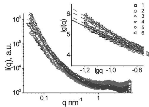
Рис. 2. МКРР дифрактограми полі(ВЕР-ко-ГМА)-графт-ПЕГ (1) та (полі(ВЕР-ко-ГМА)-графт-ПЕГ... Докс (2-6) (полімер – 10 мг/мл, [Докс] = 0,3 мг/мл (2); 0,4 мг/мл (3); 0,5 мг/мл (4); 0,6 мг/мл (5); 1,4 мг/мл (6)) (на вносці – лінійна ділянка дифрактограми). Суцільні лінії відображають собою лінійну апроксимацію відповідно до концепції масштабування
