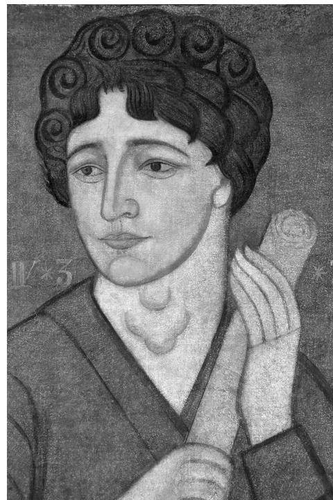
Іл. 5. М. Касперович (?). Жіночий портрет. Фрагмент (верхня частина зображення) у видимому світлі. (Фото В. Майбороди)
