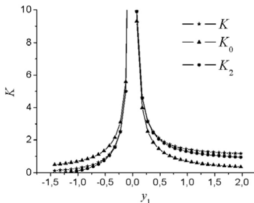
Рис. 1. Порівняння точного і наближених значень коефіцієнта підсилення першого зображення джерела (лінза Чанг-Рефсдала з \gamma = 0.3 )
