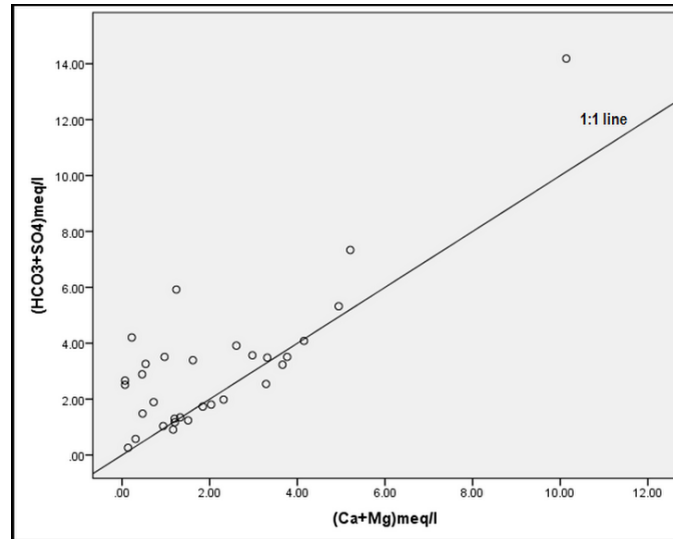
Fig. 6. \text{Ca}^{2+}+\text{Mg}^{2+} vs \text{HCO}_3^- + \text{SO}_4^{2-}
