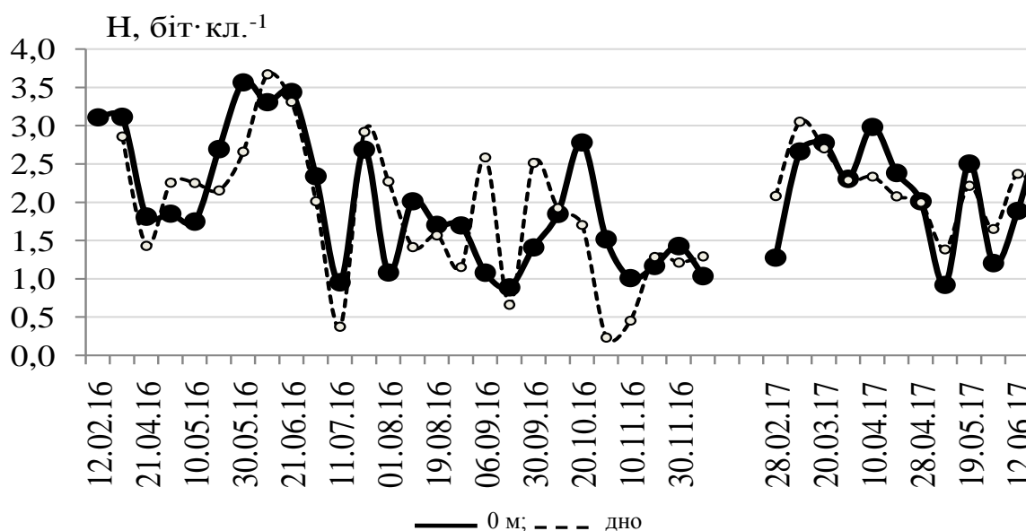
Рис. 9 – Сезонні зміни індексу Шенона (H) в поверхневих та придонних шарах води на станції (МНBS-R) в Одеській затоці в 2016–2017 рр.
