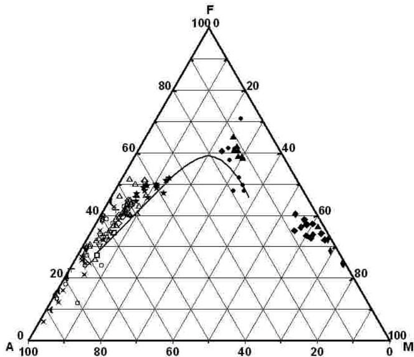
Рис. 3. Положення порід октябрського комплексу на діаграмі AFM ( \text{Na}_2\text{O}+\text{K}_2\text{O} - 0,9 \text{Fe}_2\text{O}_3+\text{FeO} - \text{MgO} ). Лінія розділу полів толейтової і валнисто-лужної серій за Ірвіном і Барагаром. Позначення ті ж, що й на рис. 1.
