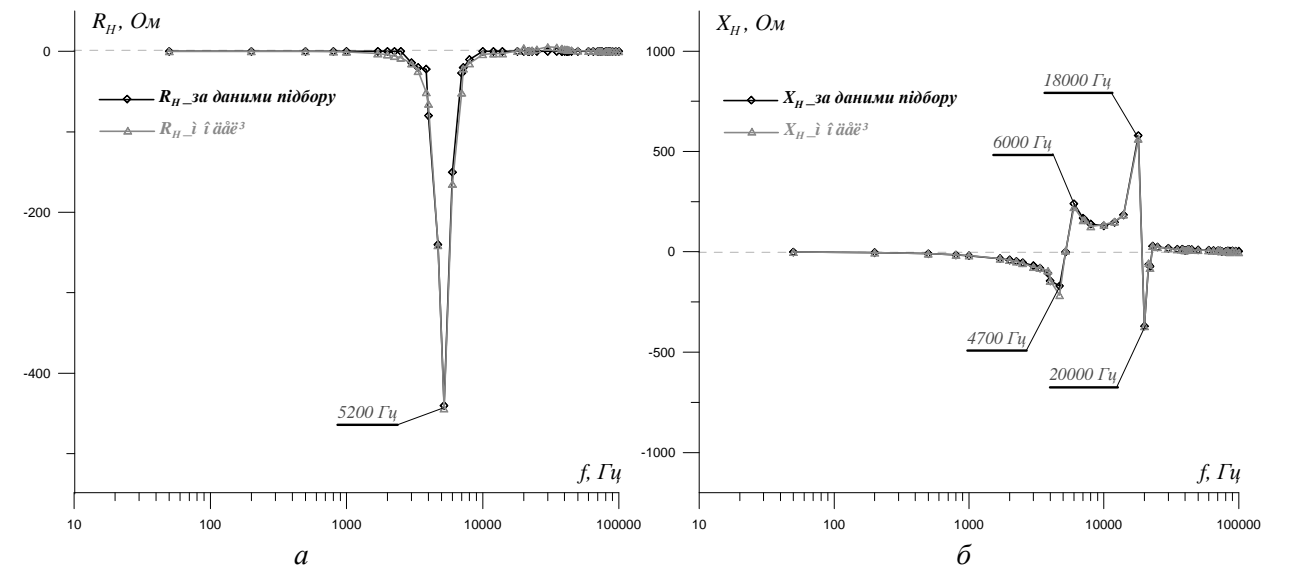
Рис. 8. Результати підбору на моделі значень модуля Z_H за даними результатів дослідів за схемою рис. 4, б та дослідів КЗ НОМ-10: а – активна складова повного опору Z_H ; б – реактивна складова повного опору Z_H
