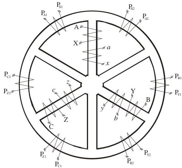
Рис. 5. Схематичне розміщення обмоток фаз і додаткових підмагнічувальних обмоток на магнітній системі
