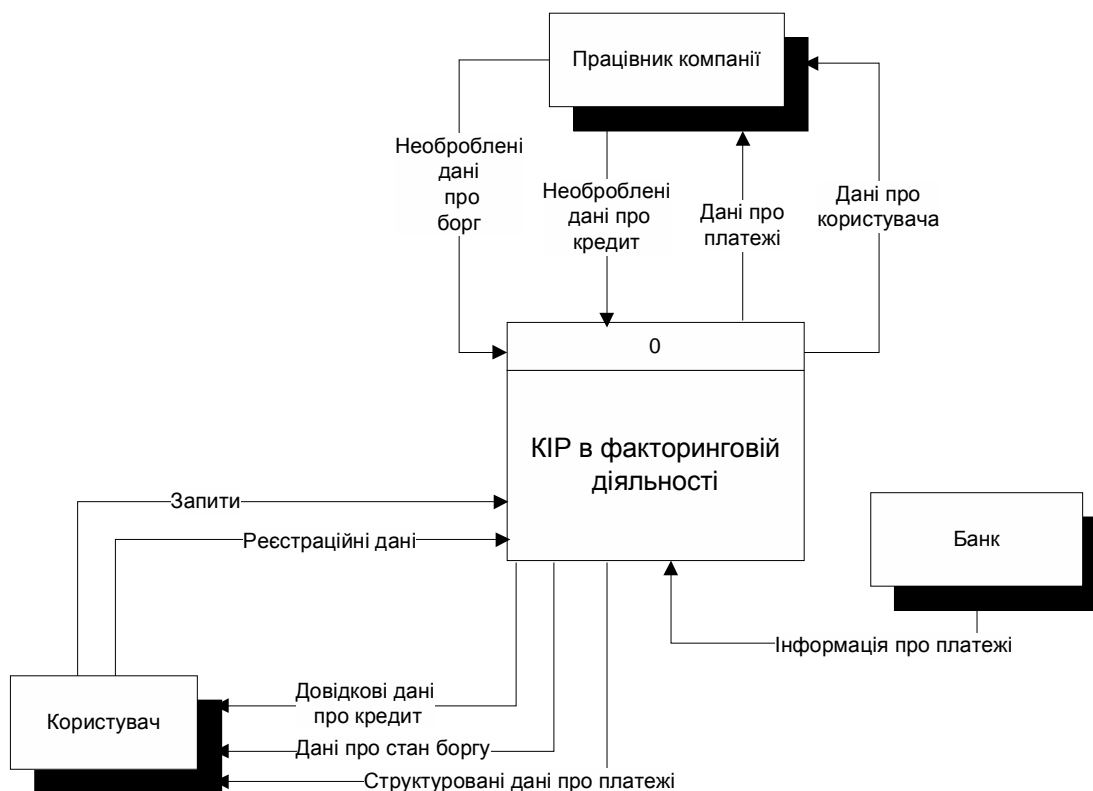
Рис. 2. Контекстна діаграма “Консолідація інформації в факторинговій діяльності”
