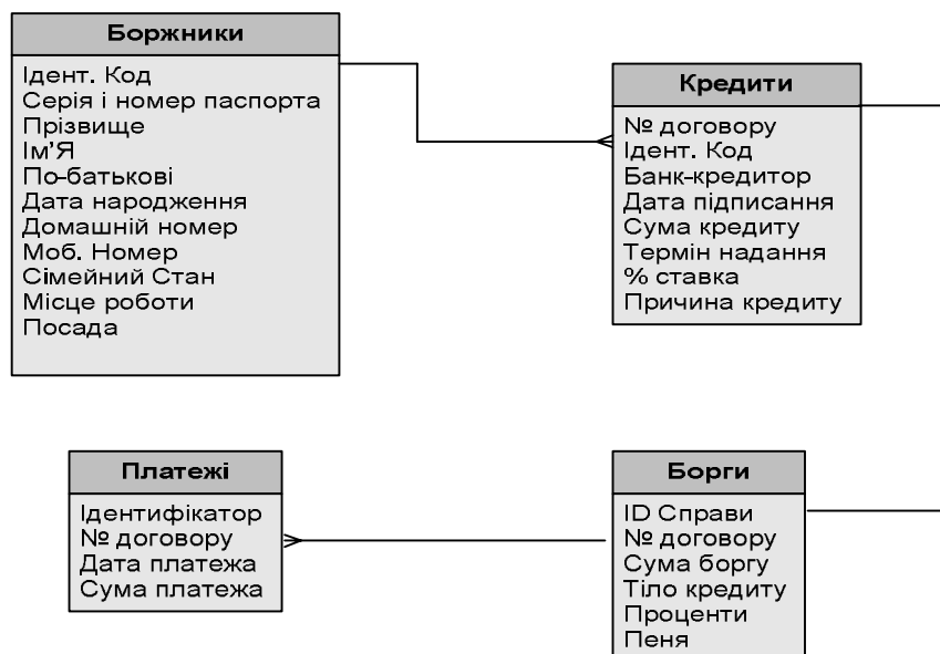
Рис. 7. ER-діаграма бази цих боргів
