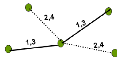
Рис. 3. Частотне планування радіорелейних каналів
