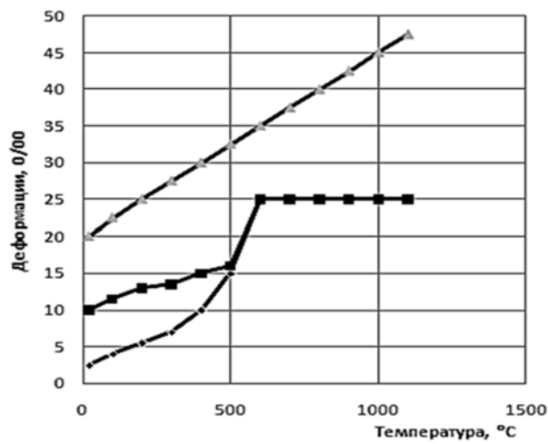
Рис. 6. Залежність деформацій \epsilon_{cu, \theta} ( \epsilon_{cl, \theta} ), \epsilon_{cu1, \theta} і \epsilon_{ce, \theta} від температури
