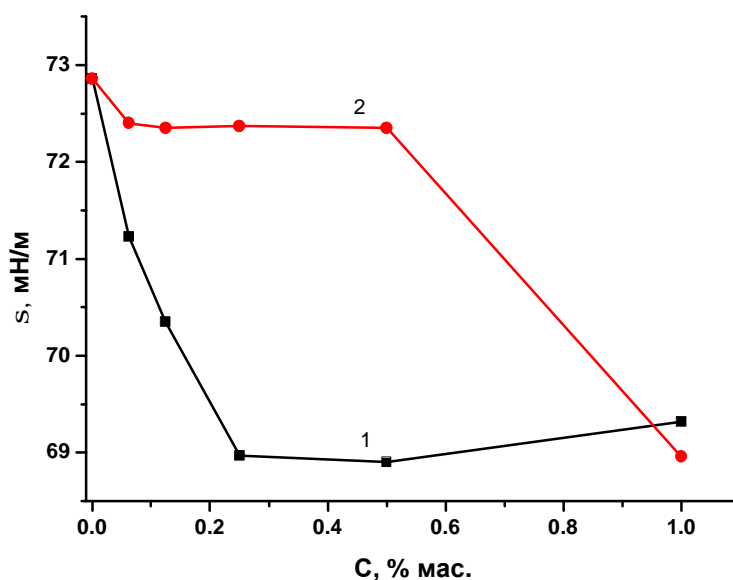
Рис. 1. Залежність поверхневого натягу за температури 20^\circ\text{C} водних розчинів полімерів від їх концентрацій: 1 – водний розчин ПВП; 2 – водний розчин ПАА
