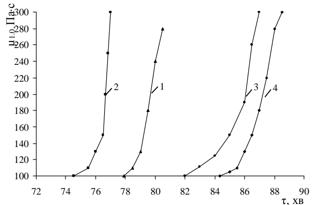
Рис. 2. Кінетичні залежності в'язкості за методом Брукфільда поліестерних композицій під час тверднення в присутності модифікатора (2 % мас.): 1 – нікель-силікатний; 2 – ПВХ; 3 – немодифікована поліестерна смола; 4 – цинк-силікатний. Швидкість зсуву 1 \text{ сек}^{-1}
