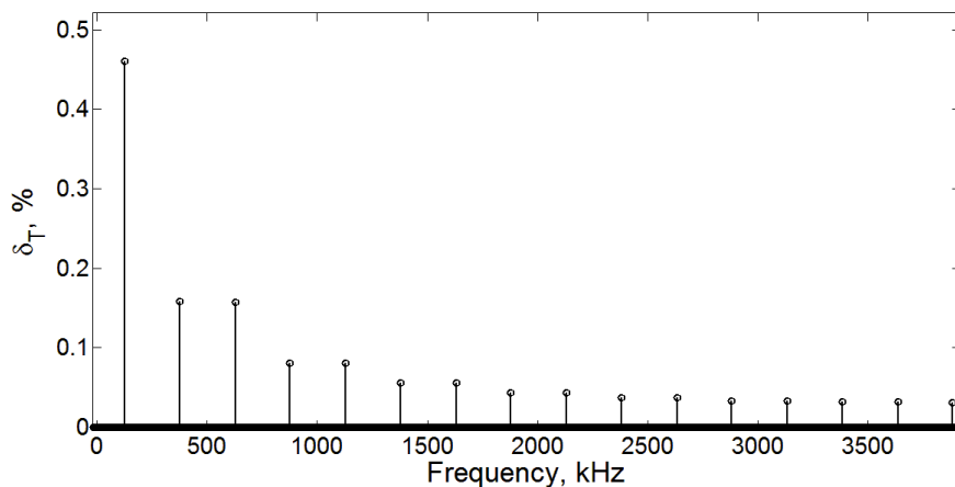
Рис. 2. Похибка від усікання коду акумулятора фази в часовій (а) та частотній областях (б)
