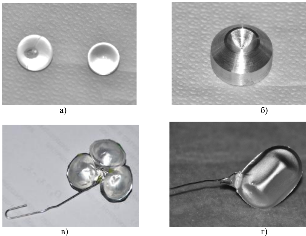
Рис. 4. Акустичні лінзи:
