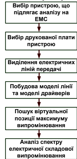
Рис 2. Порядок дослідження плат на EMC
