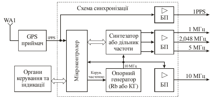
БП – буферний підсилювач; Rb – рубідієвий генератор; КГ – кварцовий генератор (ОСХО) Рис. 3. Структурна схема синхрогенератора з рубідієвим стандартом
