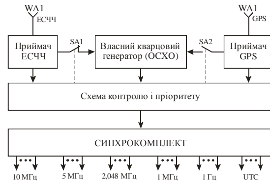
Рис. 7. Комбінований синхрокомплект
