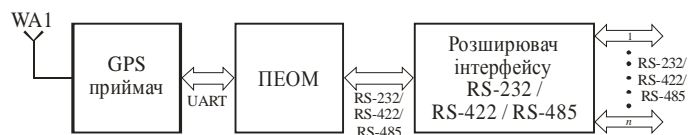
Рис. 5. Структурна схема пристрою синхронізації за протоколом NMEA 0183
