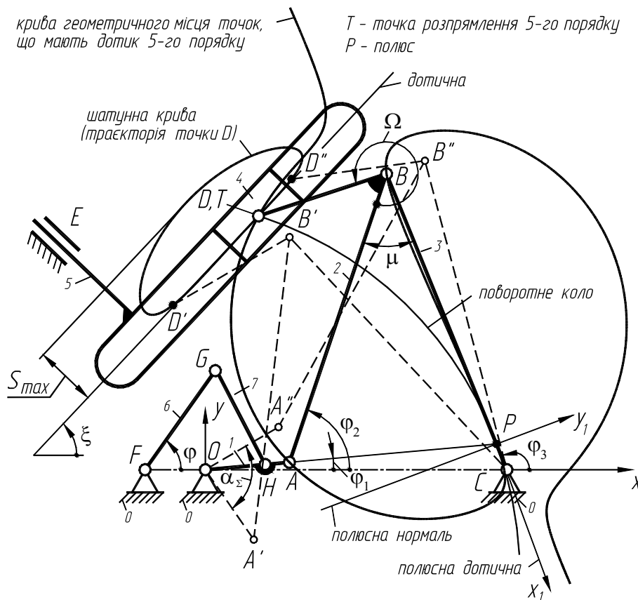
Рис. 1. Важільний восьмиланковий механізм із зупинкою вихідної ланки
