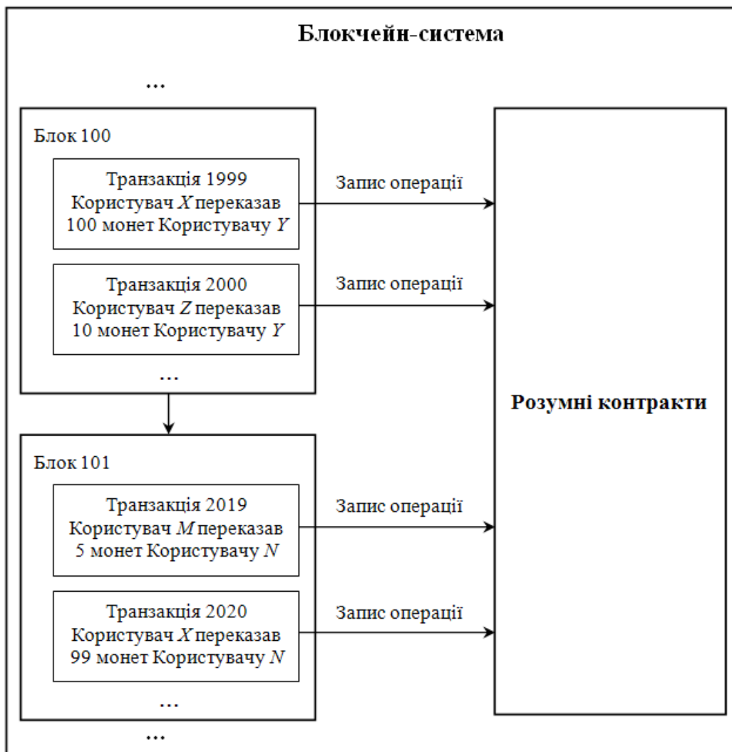
Рис. 2. Опрацювання транзакцій всередині блокчейн-системи
