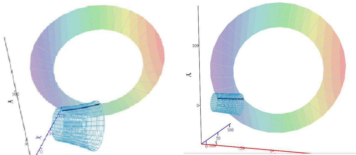
Рис. 2. Формоутворення заправленим торцем круга по рядках на поверхні деталі при різних значеннях відстані між осями
