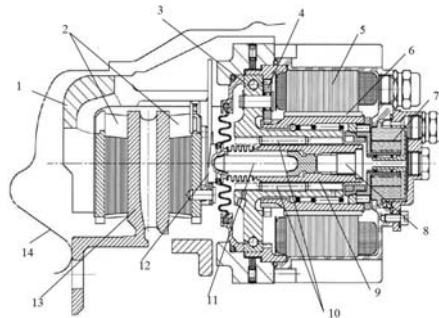
Рис. 2 – Конструкція виконавчого елемента; 1 – супорт; 2 – гальмівні колодки; 3 – центральний підшипник; 4 – планетарний механізм; 5 – статор; 6 – ротор/гайка; 7 – вирішальний пристрій; 8 – датчик сили; 9 – шпindelь; 10 – планетарні ролики; 11 – натискний шток; 12 – підтримка колодки; 13 – гальмівний диск; 14 – корпус.
