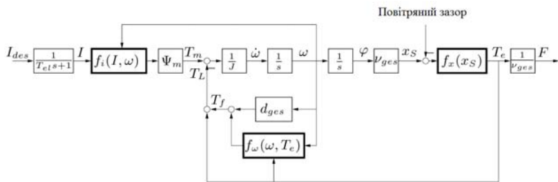
Рис. 3 – Математична модель електромеханічного гальма; d_{ges} - Загальна в'язкого тертя; f_i(I, \omega) - зворотній зв'язок двигуна; f_x(x_S) - функція передачі між кутом обертання шпинделя і притисної сили; f_\omega(\omega, T_c) - функція передачі між кутом обертання крутного моменту і тертя; F - сила притискання; J - момент інерції; T_c - крутний момент; T_f - момент тертя; T_L - доступний момент навантаження T_L = T_c + T_f ; T_m - електричний крутний момент; T_{el} - електрична постійної часу двигуна; x_S - позиція шпинделя; \nu_{ges} коефіцієнт пропускання; \varphi - кут обертання; \Psi_m - магнітний потік; \omega - кутова швидкість.
