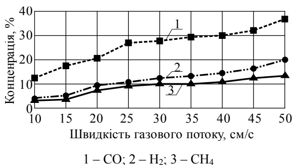
Рис. 1. Концентрація горючих газів від швидкості газового потоку.
