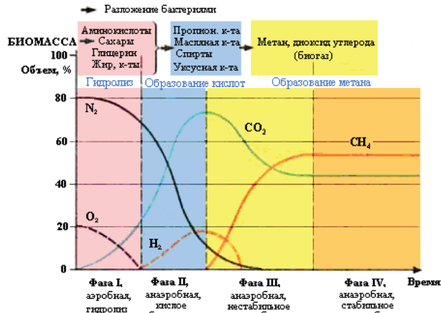
Рис. 2. Стадии разложения органических отходов
