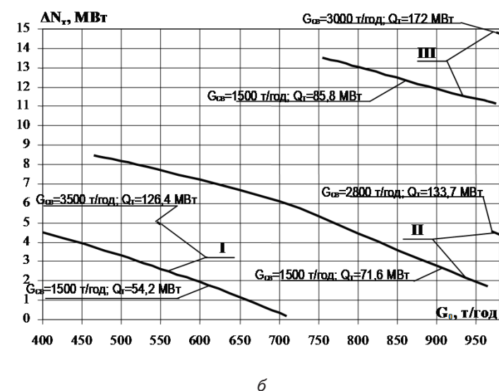
Рис. 7. Зміна потужності турбіни на теплофікаційному режимі в залежності від витрати свіжої пари: а – турбіна Т-100/120-130; б – турбіна Т-250/300-240; I – t_{3н}=+10\text{ }^\circ\text{C} , t_1=46\text{ }^\circ\text{C} , t_2=77\text{ }^\circ\text{C} ; II – t_{3н}=0\text{ }^\circ\text{C} , t_1=46\text{ }^\circ\text{C} , t_2=87\text{ }^\circ\text{C} ; III – t_{3н}=-5\text{ }^\circ\text{C} , t_1=51\text{ }^\circ\text{C} , t_2=100\text{ }^\circ\text{C} – режими роботи турбоустановок
