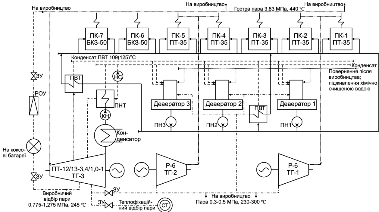
Рис. 1. Принципова тепла схема ТЕЦ ТОВ «Ясинівський КХЗ»
