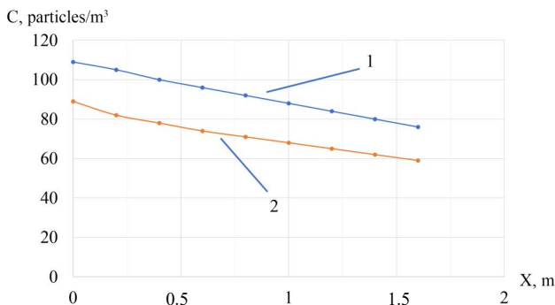
Fig. 7. The number of dust particles that «settled» on the vertical «sensitive» surface per day: 1 – scenario No. 1; 2 – scenario No. 2
