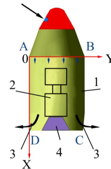
Fig. 3. Estimation scheme:
