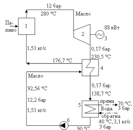
Рисунок 1 – Принципова теплова схема когенераційної установки
