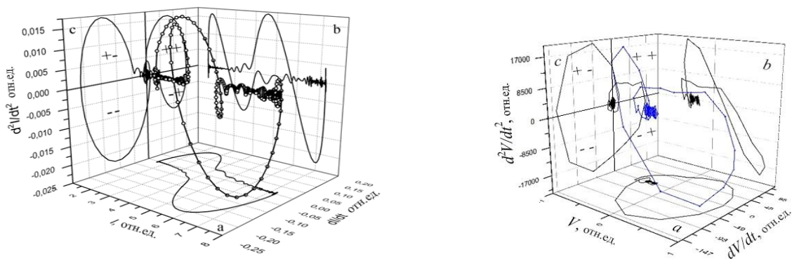
а) б) Рисунок 1 – Фотовідгук сенсора (а) і кардіосигнал (б) як траєкторії динамічних подій в просторі (стан-швидкість-прискорення), а також ортогональні проєкції цих траєкторій – сигнатури: а) I(t) - dI/dt ; б) I(t) - d^2I/dt^2 ; в) dI/dt - d^2I/dt^2 , (на рис. 1 б представлено аналогічні сигнатури кардіоциклу)
