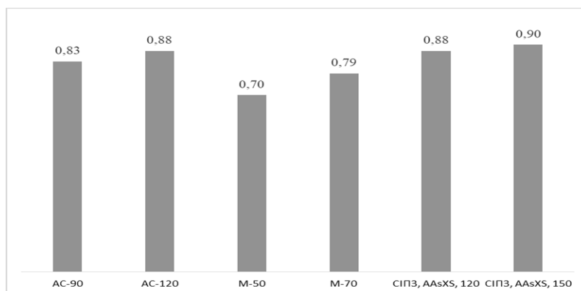
Рис. 5. Напряга у відносних одиницях при струмі 35,29 А.
