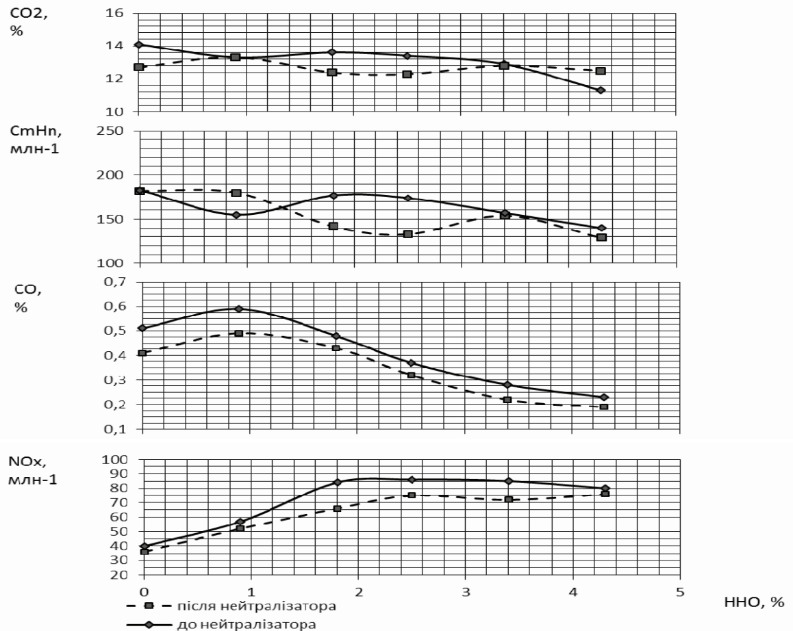
Рисунок 6. Вплив добавки суміші H 2 /O 2 на склад відпрацьованих газів
