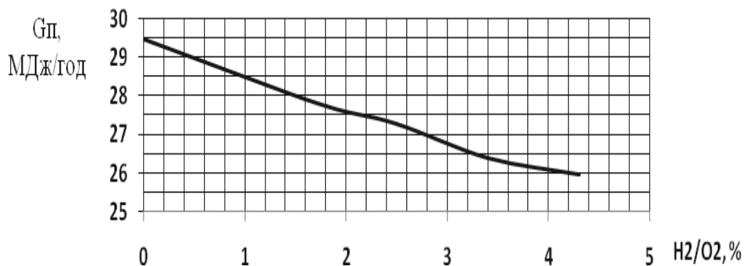
Рисунок 3. Витрата палива в тепловому еквіваленті при додаванні газу H_2/O_2 ( n=900 хв -1 )
