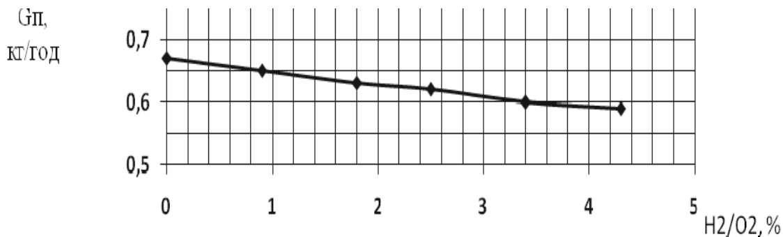
Рисунок 2 - Залежність годинної витрати палива від величини добавки H_2/O_2 ( n = 900 \text{ хв}^{-1} )
