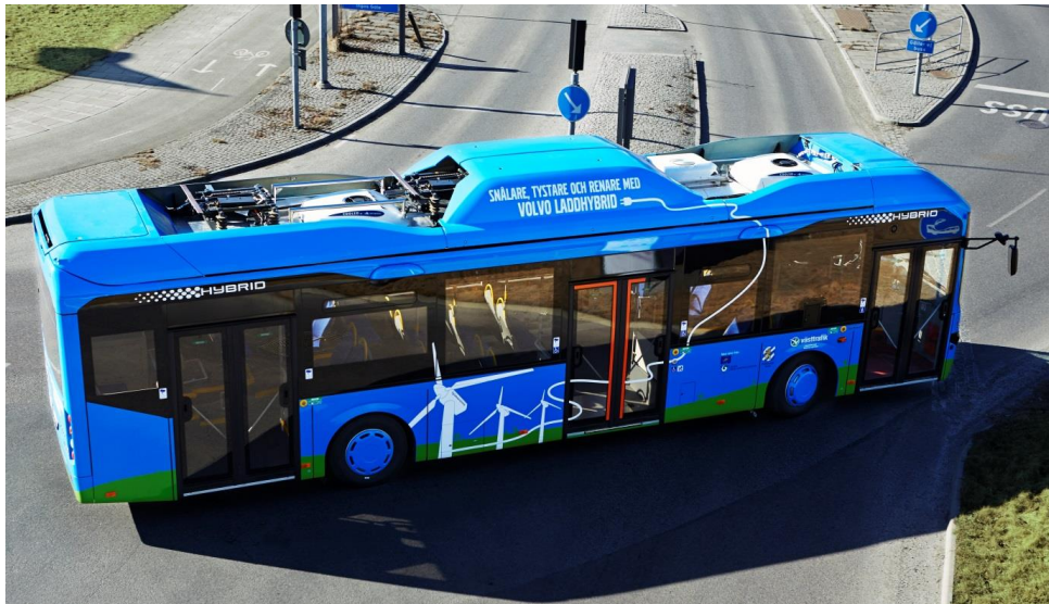
Rys. 5. Autobus szybko ładowany na przystankach autobusowych przez automatyczny system połączeń montowany na dachu autobusu ACS (Automatic Roof-Top Connection System)[2, 5]
