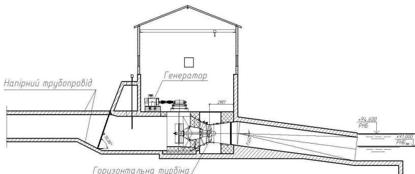
Рис. 7. Горизонтальна турбіна SINK Hydro-Energy k.s, Чехія
