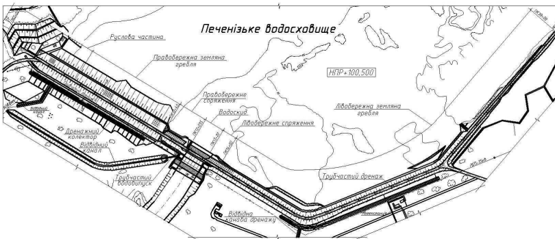
Рис. 2. План Печенізького гідровузла
