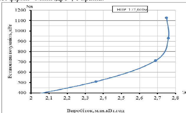
Рис. 1. Залежність середньорічної виробітки від встановленої потужності ГЕС в м. Житомирі (при встановленні двох гідроагрегатів)
