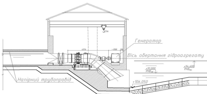
Рис. 5. Прямоточна турбіна Т-90, ТОВ «Мінігідро», Україна
