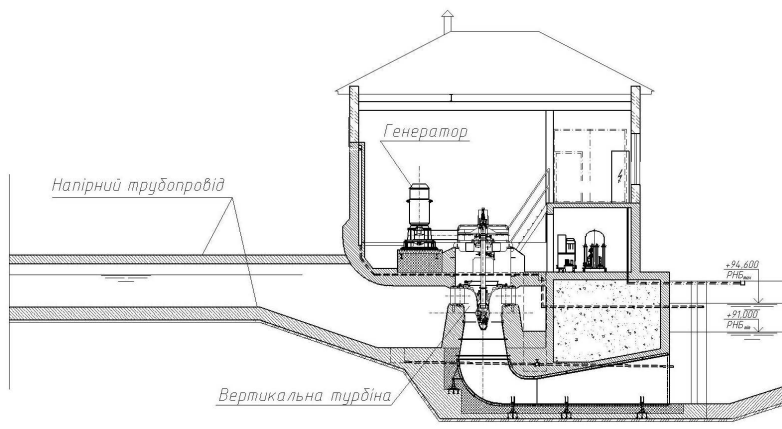
Рис. 4. Вертикальна турбіна KAPLAN KVK1900R4 фірми MAVEL, Чехія
