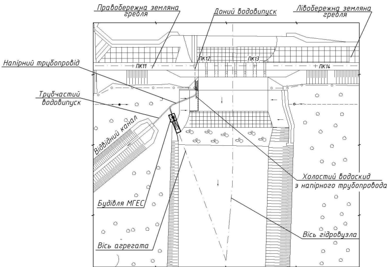
Рис. 3. План розміщення МГЕС в складі Печенізького гідровузла
