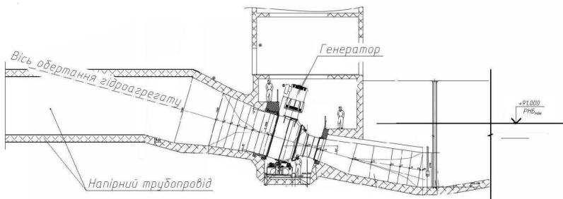
Рис. 6. Турбіна KRT 5-1700, фірми Andritz Hydro, Австрія
