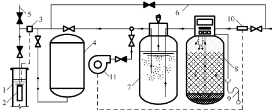
Рис. 1. Схема знезалізнення води з напірним фільтром та аерацією компресором: 1 – свердловина; 2 – занурений насос; 3 – реле тиску; 4 – гідроакумулятор; 5 – поливальна труба; 6 – обвідна лінія; 7 – аераційна колона з повітровідділювачем; 8 – напірний знезалізнювальний фільтр з клапаном управління; 9 – каналізаційна труба; 10 – водолічильник з імпульсним виходом; 11 – компресор
