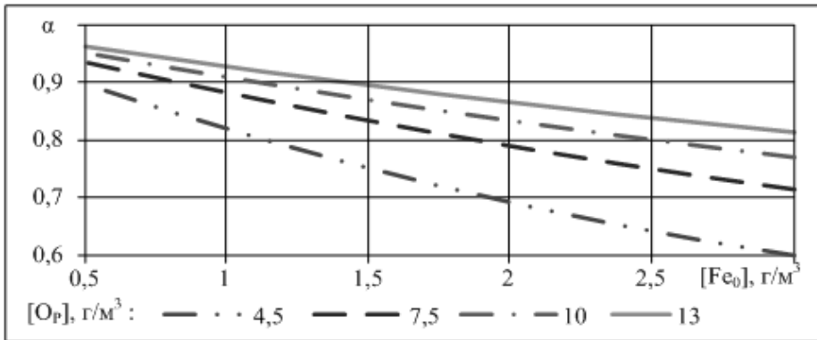
Рис. 3. Залежність коефіцієнта рециркуляції води \alpha від концентрації заліза в підземній воді [Fe_0] та концентрації розчиненого кисню в рециркуляційній трубі [O_2]
