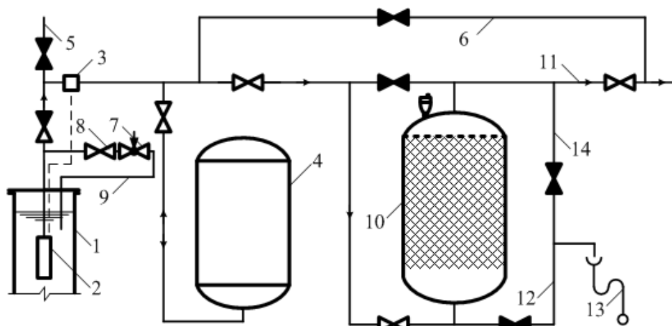
Рис. 2. Схема знезалізнення води з напірним пінополістирольним фільтром та аерацією на рециклі: 1 – свердловина; 2 – занурений насос; 3 – реле тиску; 4 – гідроаккумулятор; 6 – обвідна лінія; 7 – ежекційний аератор; 8 – регулювальний вентиль; 9 – рециркуляційний трубопровід; 10 – напірний пінополістирольний фільтр; 11 – трубопровід знезалізненої води; 12 – промивний трубопровід; 13 – каналізаційна труба; 14 – трубопровід скиду першого фільтрату
