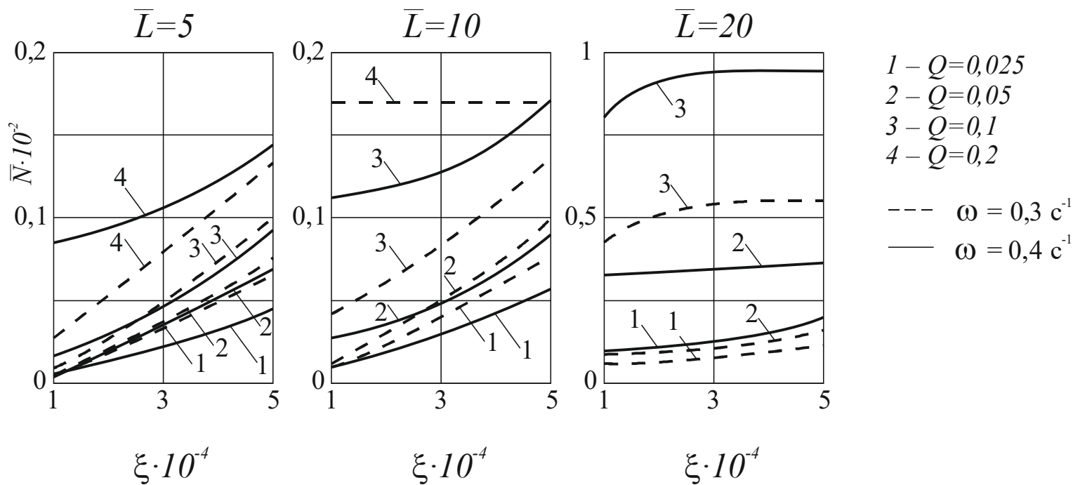
Рисунок. Графіки \bar{N} = f(\xi) в межах області РК застосування фільтра ССФ-200
