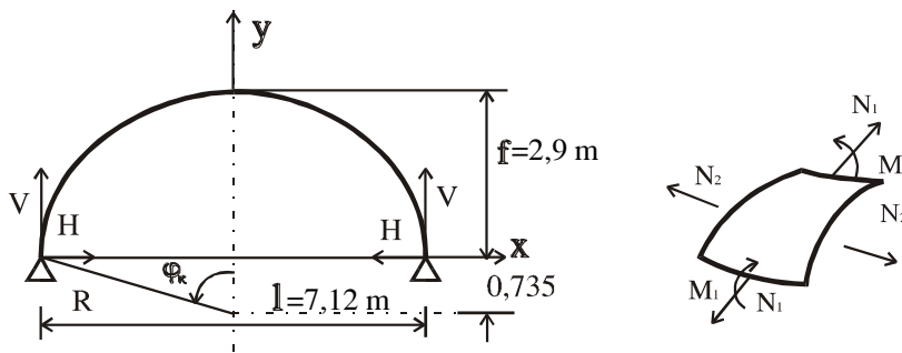
Рис. 1 Купол: а) геометрия сечения; б) схема усилий
