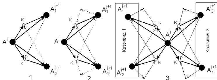
Рис.5 Образование квазивидов и саморепликация 1,2 – схемы образования квазивидов кластеров из одного и того же субстрата, 3 – явление саморепликации квазивидов кластеров
