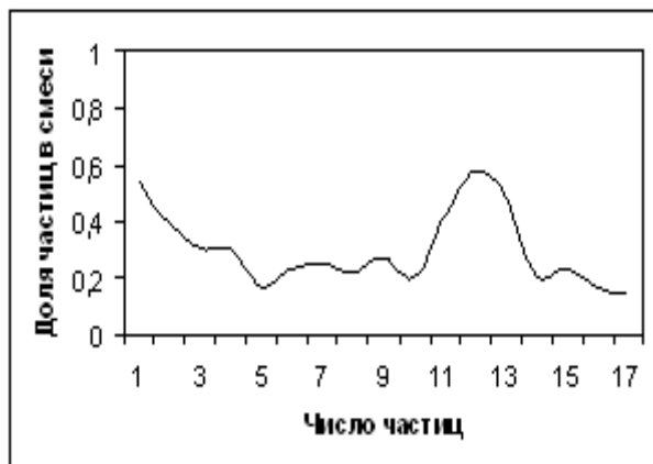
Рис.2. Качественный вид распределения кластеров по числу частиц.
