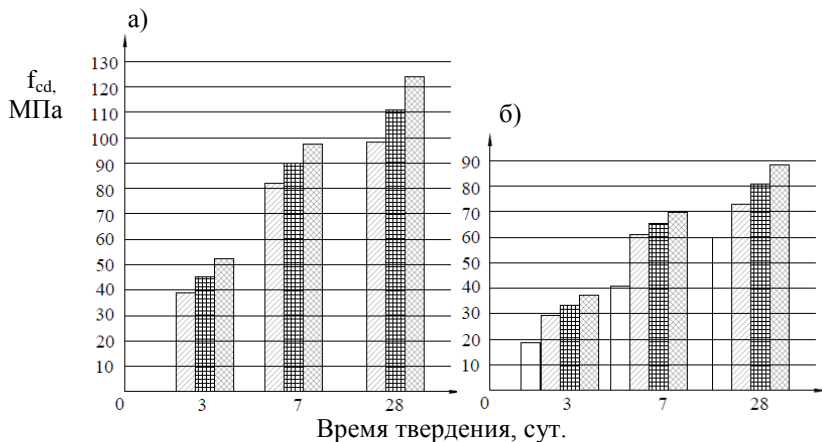
Рис. 1. Влияние концентрации микрокремнезема на f_{cd} бетона (расход вяжущего 550 \text{ кг/м}^3 , S_{уд} = 500 \text{ м}^2/\text{кг} );
