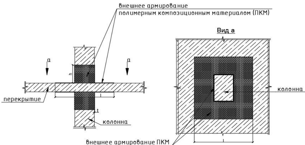
Рис. 3. Внешнее армирование углепластиковым холстом соединения перекрытия и колонны
