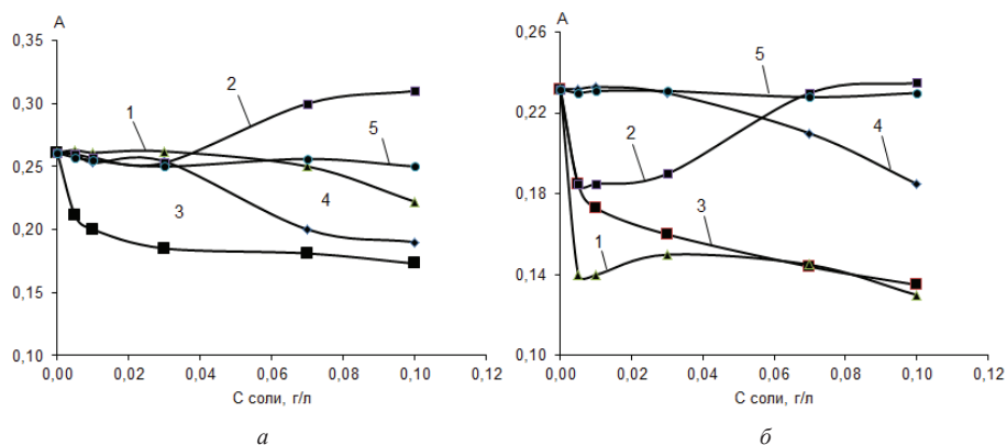
Рис. 7. Зависимость оптической плотности ассоциата БФС-FO4990 в присутствии неорганических солей. \lambda = 590 нм (а), 437 нм (б), pH = 3,6, C_{\text{БФС}} = 2 \cdot 10^{-3} моль/л, l = 1 см.
