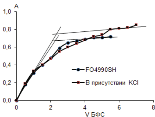
Рис. 8. Кривые титрования полимера FO4990SH в отсутствии и присутствии 65 мг/л KCl. \lambda = 590 нм, pH = 3,6, C_{\text{БФС}} = 5 \cdot 10^{-5} моль/л, l = 5 см.
