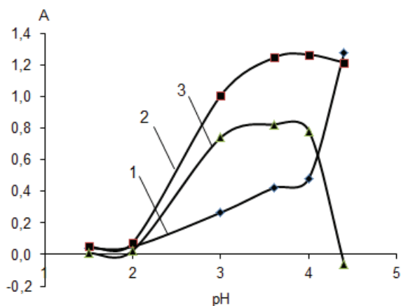
Рис. 5. Зависимость оптической плотности БФС (1), БФС-ФО (2) и \Delta A от рН (3). C_{\text{БФС}} = 2 \cdot 10^{-5} моль/л, C_{\text{ФО}} = 12 мг/л, l = 1 см
