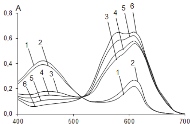
Рис. 4. Спектры поглощения ассоциата БФС-КПАА при различной плотности заряда полиэлектролита. Плотность заряда: 1 – 5%, 2 – 5=10%, 3 – 30%, 4 – 55%, 5 – 70%, 6 – 95%. рН = 3,6, C_{\text{БФС}} = 2 \cdot 10^{-5} моль/л, C_{\text{FO}} = 12 мг/л, l = 1 см
