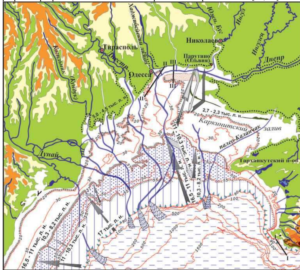
Рис. 1. Схематическая карта развития северо-западного шельфа Черного моря в новозвквинско-голоценовое время (18–17 тыс. л. н. — до наших дней).
