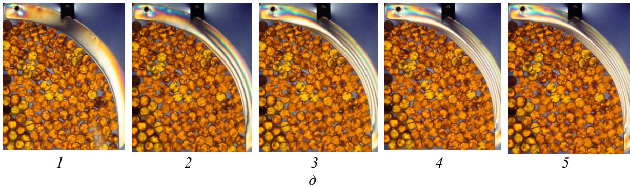
Рис. 7. Фотограми процесу виникнення напружень від навантаження на задніх стінках ковшів скреперів: а – традиційна задня стінка ; б – в – г – д – – задні стінки ковшів скреперів з напівкруглим днищем; 1 – 5 – фотограми напруження задніх стінок ковшів скреперів
