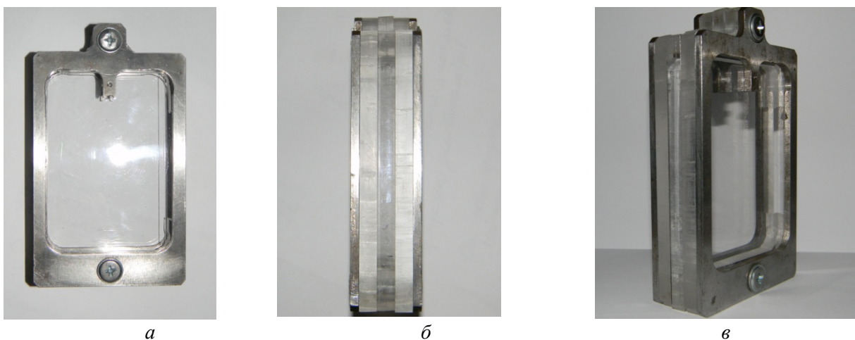
Рис. 5. «Прозорий» контейнер у зборі: а – вигляд спереду; б – вигляд збоку; в – аксонометрична проекція
