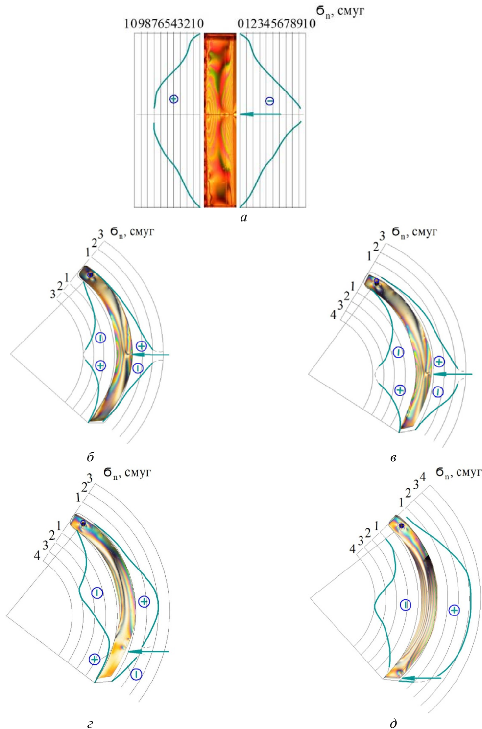
Рис. 6. Isochroms (смуги) й епюри напружень у моделях задніх стінок скрепера: а – традиційна задня стінка ; б – , в – , г – , д – – задні стінки ковзів скреперів із напівкруглим днищем
