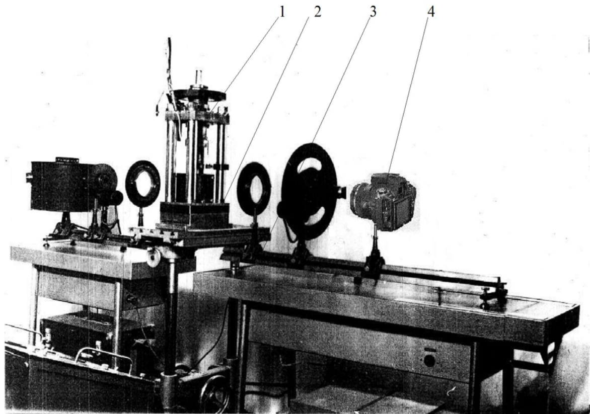
Рис. 4. Загальний вигляд станда для дослідження напружень поляризаційно-оптичним методом з реєструвальною апаратурою: 1 – лабораторний прес; 2 – стіл ПС-1; 3 – поляризаційно-проекційна установка ППУ-7; 4 – кінокамера Nikon
