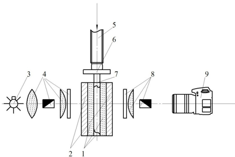
Рис. 3. Схема стэнда для дослідження напружень поляризаційно-оптичним методом: 1 – скляні блоки; 2 – контейнер; 3 – лампа; 4, 8 – вузли поляризатора й аналізатора ППУ-7; 5 – гвинт преси; 6 – прижимна частина преси; 7 – насадка інструмента; 9 – фотоапарат
