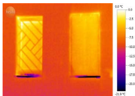
Рис. 3. Термограмма фрагмента ограждающей конструкции с однокрамным оконным блоком и с установкой дополнительной оконной рамы из поликарбоната (4 мм)
