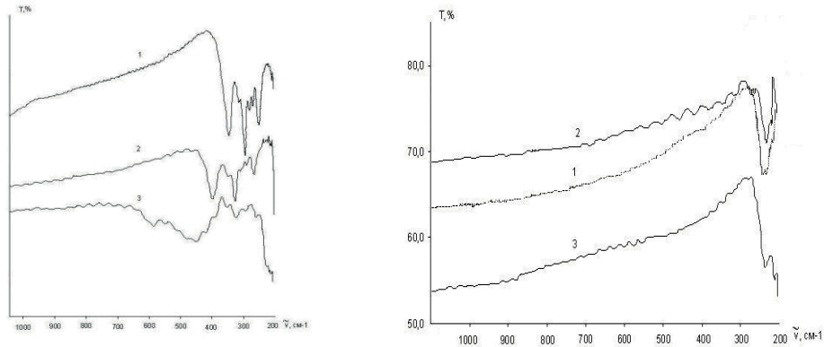
Рис. 2. ИК-спектры пропускания систем: \text{EuIn}_2\text{S}_4\text{-Ge} (а); \text{EuIn}_2\text{Se}_4\text{-Ge} (б): 1 — халькогенид; 2 — композит; 3 — остаток после испарения
