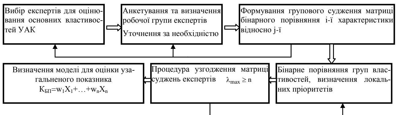
Рис. 1. Процедура визначення вагового внеску основних груп властивостей в узагальнений показник бойової ефективності ( K_{БП} – коефіцієнт бойового потенціалу; w_1 \dots w_n ваговий коефіцієнт кожної з виділених груп властивостей; X_1 \dots X_n – виділені групи властивостей; \lambda_{\max} – максимальне власне значення матриці бінарних порівнянь; n – порядок матриці)
