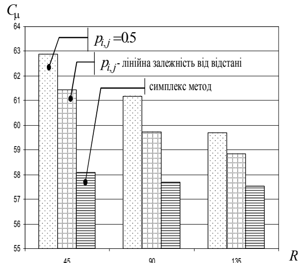
Рис. 3. Залежність математичного сподівання вартості топології від розміру популяції
