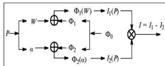
Рис. 2. Послідовність перетворення сигналів диференціального ВОДД відбивного типу
