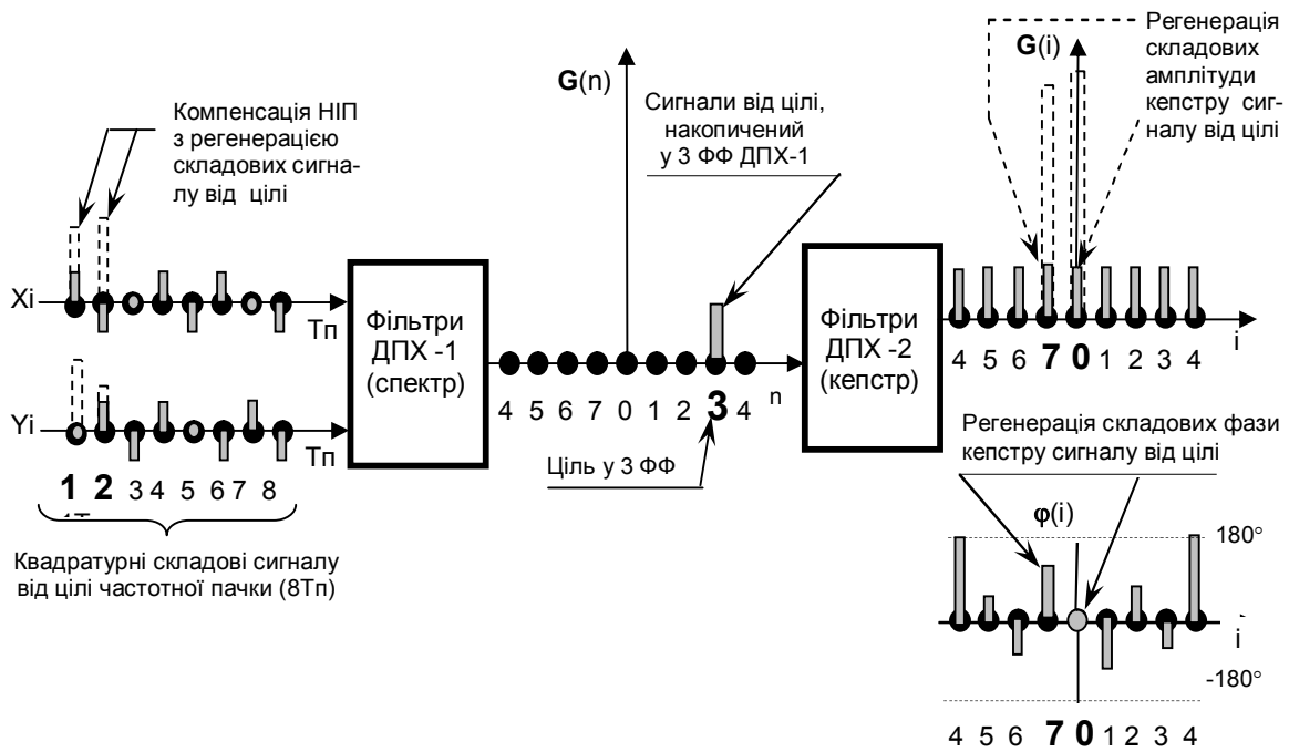
Рис. 3. До пояснення принципу регенерації складових кепстру сигналів від цілі для випадку уражень імпульсами НІП дискрет дальності у 1T_p та 2T_p
