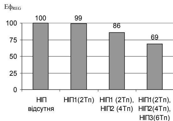
Рис. 5. Залежності показника ефективності компенсатора НІП з регенерацією E_{f_{REG}} від кількості уражень НІП
